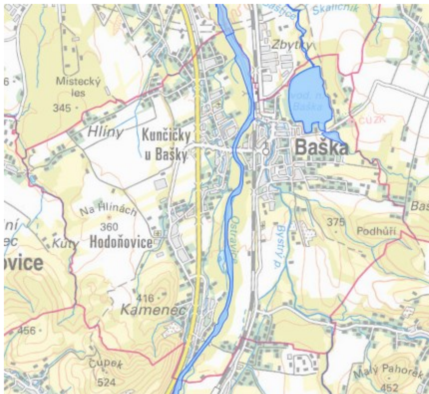
Obrázek 10 – Záplavové území 5leté vody na území obce Baška
